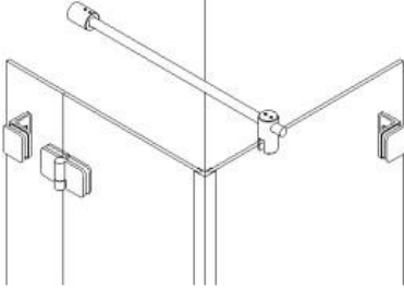
Haltestange Glas Wand 90°
