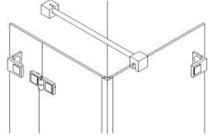
Haltestange eckig Glas Wand 90°
