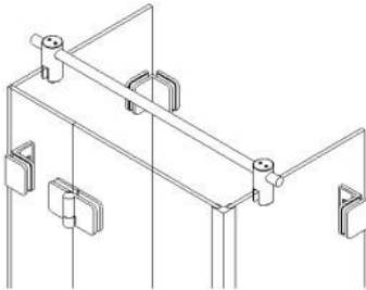
Haltestange Glas Glas 180°
