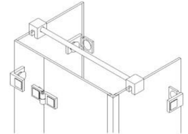
Haltestange eckig Glas Glas 180°
